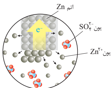
اکسایش اتم‌های روی در سطح آند
