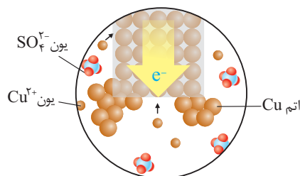
کاهش یون‌های مس در سطح کاتد
